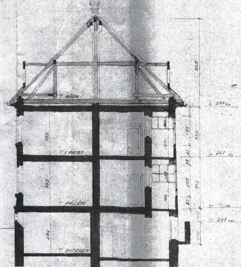
ŘEZ A-B
