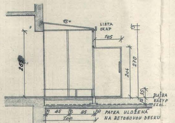
ŘEZ PŘÍSTAVKEM
