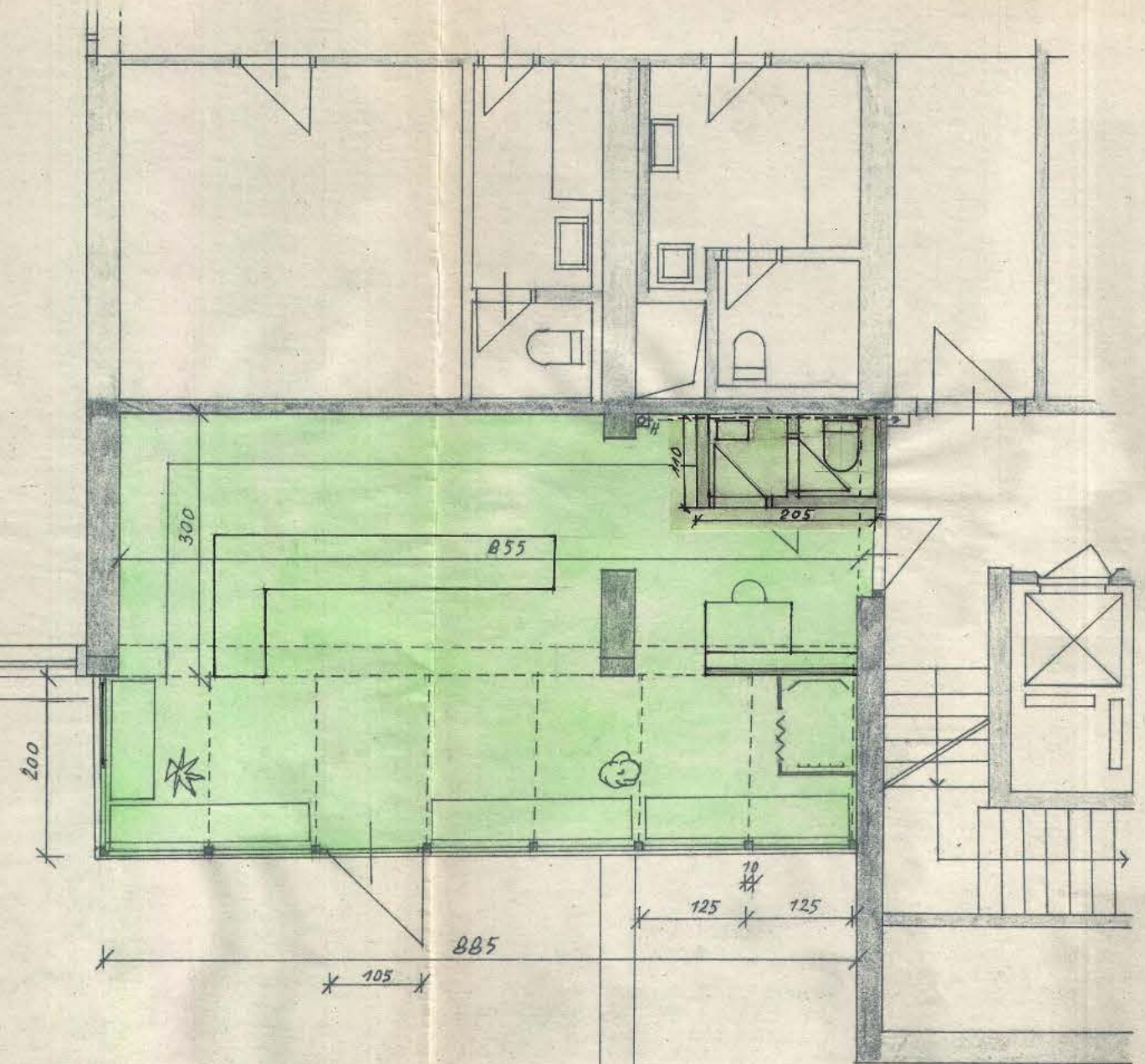
PŮDORYS OBCHODU
